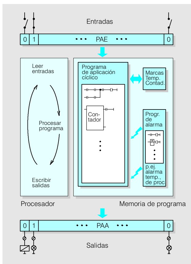
Fig. 4/9 Estructura funcional del S5-135U, S5-155U
