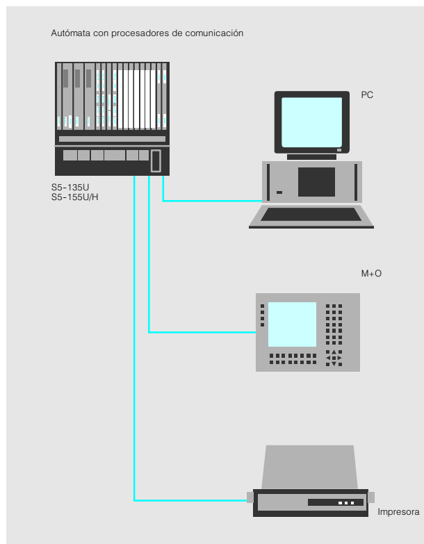
Fig. 4/11 Acoplamiento de autómatas con PC, aparatos M + O e impresoras
