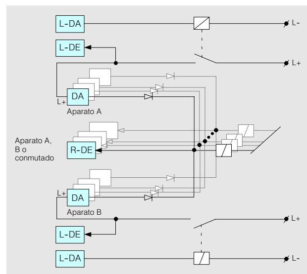
Fig. 11/10 Salida digital intermitente redundante bicanal con localización de fallos reducida
