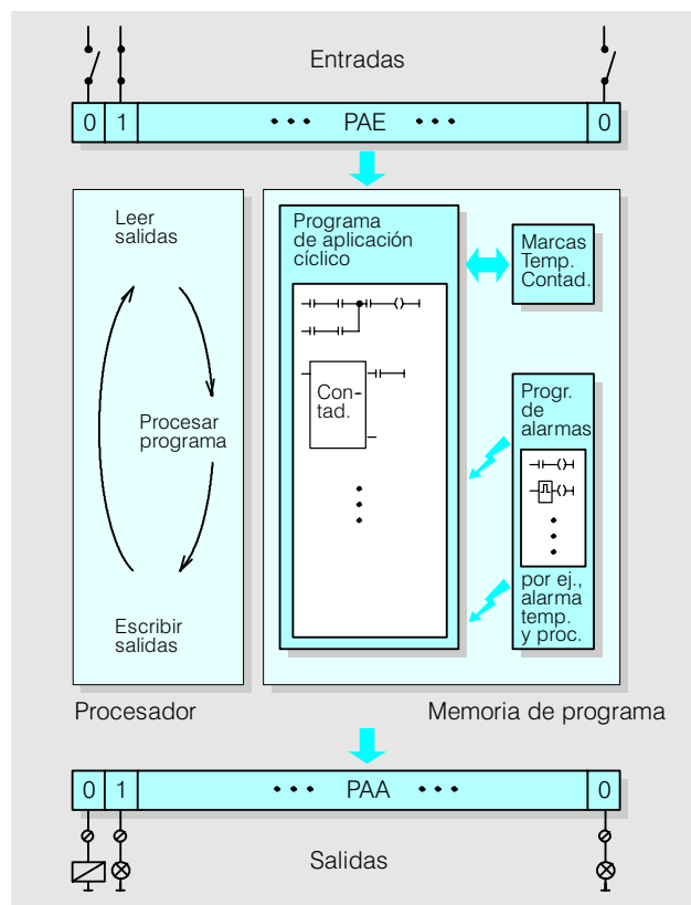
Fig. 3/4 Funcionamiento del S5-115U
