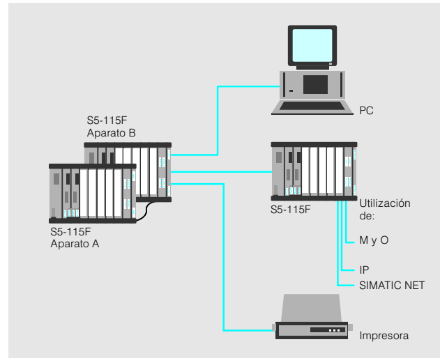
Fig. 3/22 Acoplamiento punto a punto del S5-115F con CP 523 o por el conector PG
