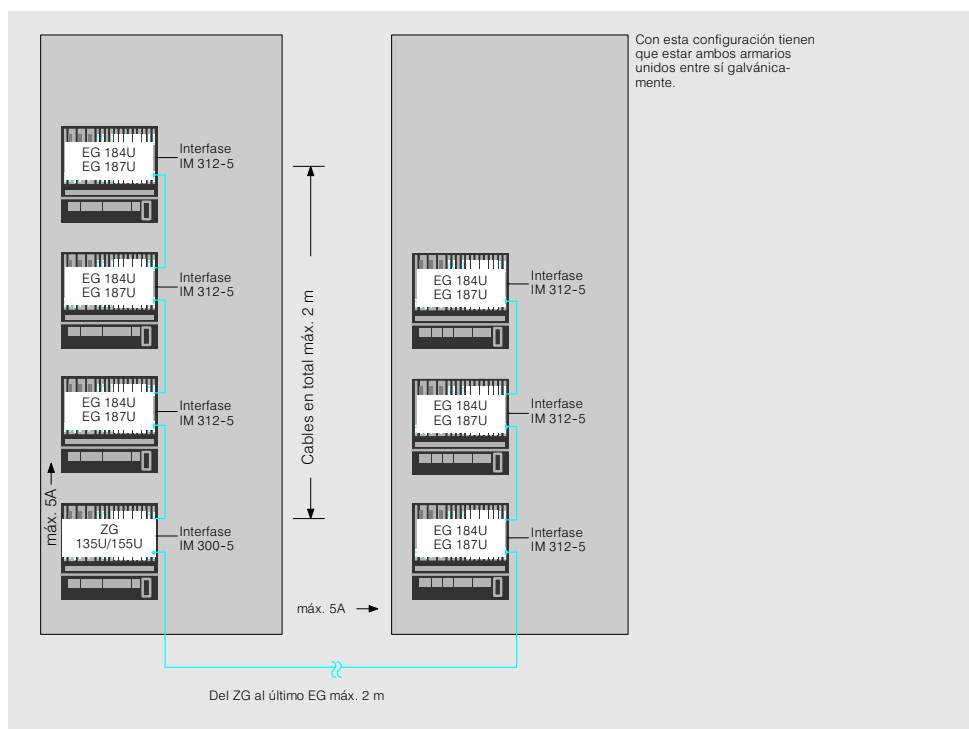
Fig. 4/49 Conexión centralizada de aparatos de ampliación sin fuente de alimentación insertada en el aparato central vía interfases IM 312-5 e IM 300-5.
