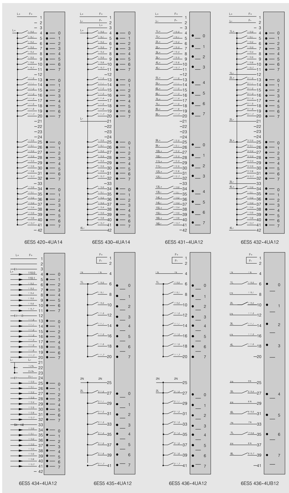
Fig. 4/23 Esquemas de conexiones de las tarjetas de entrada digitales
