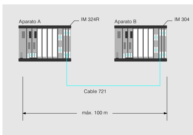
Fig. 3/37 Acoplamiento de ambos aparatos centrales
