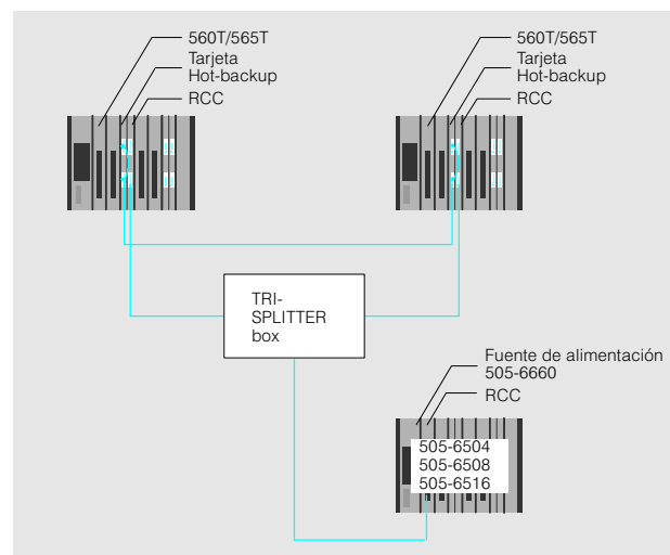
Fig. 5/2 Hot-backup con periferia monocanal
