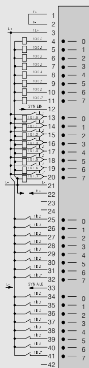
6ES5 482-4UA11
