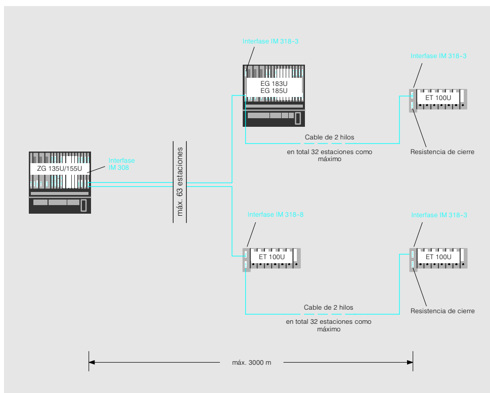
Fig. 4/55 Conexión descentralizada de aparatos de ampliación y regletas electrónicas al aparato central vía interfases IM 318 e IM 308
