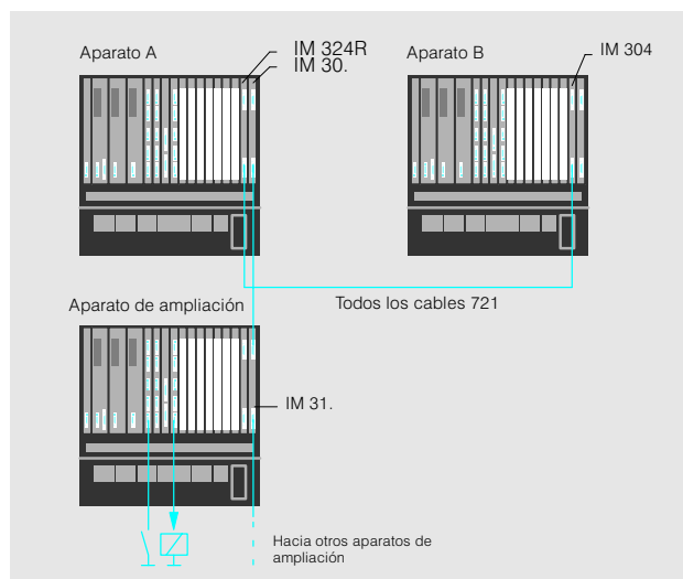
Fig. 4/14 Configuración monocanal (disponibilidad normal)
