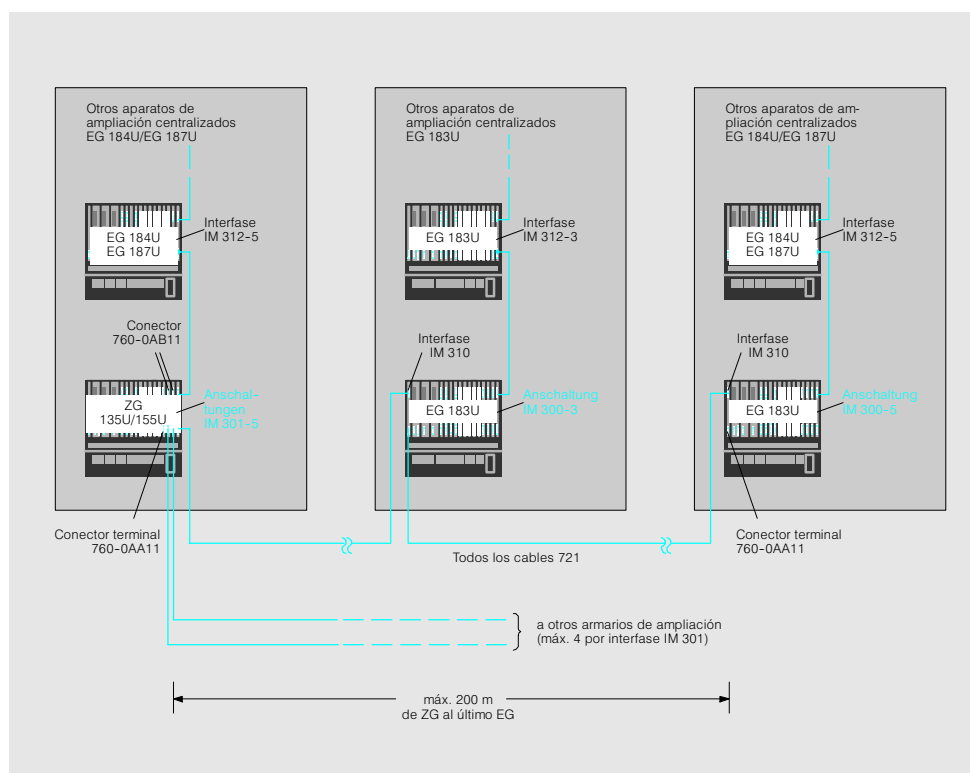
Fig. 4/51 Conexión descentralizada de EG 184U/EG 187U al aparato central vía interfases IM 310 e IM 301-5
