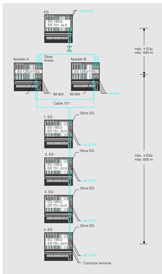
Fig. 4/57 Configuración conmutación descentralizada de tarjetas periféricas
