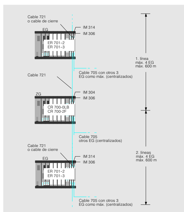
Fig. 3/41 Configuración de aparatos descentralizada
