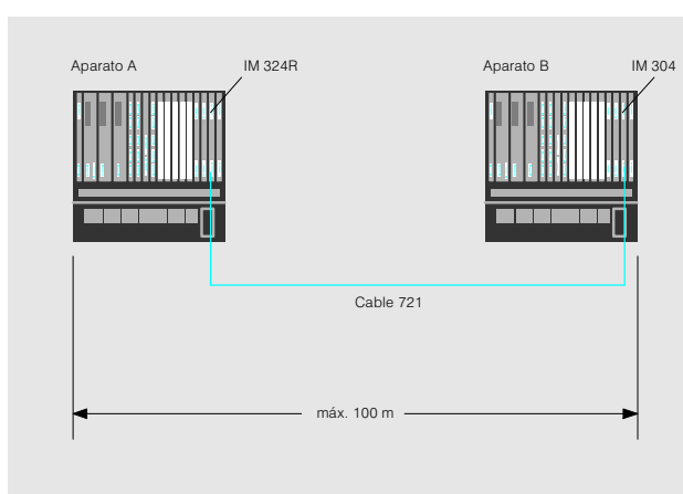
Fig. 4/56 Acoplamiento de ambos aparatos centrales
