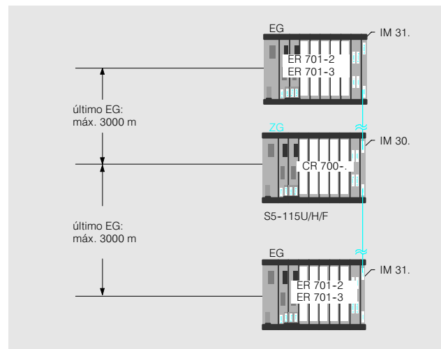
Fig. 3/3 Conexión descentralizada de aparatos de ampliación
