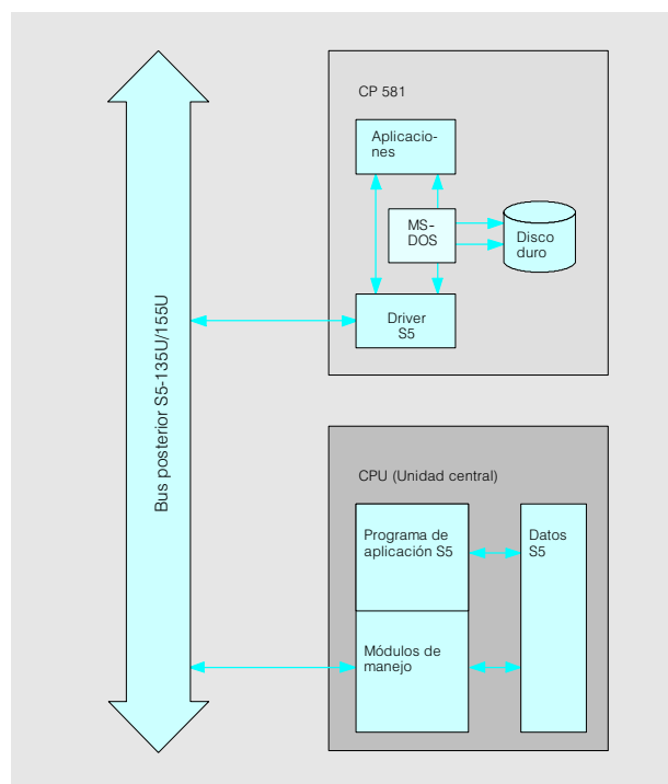
Fig. 4/44 Intercambio de datos entre CP 581 y CPU
