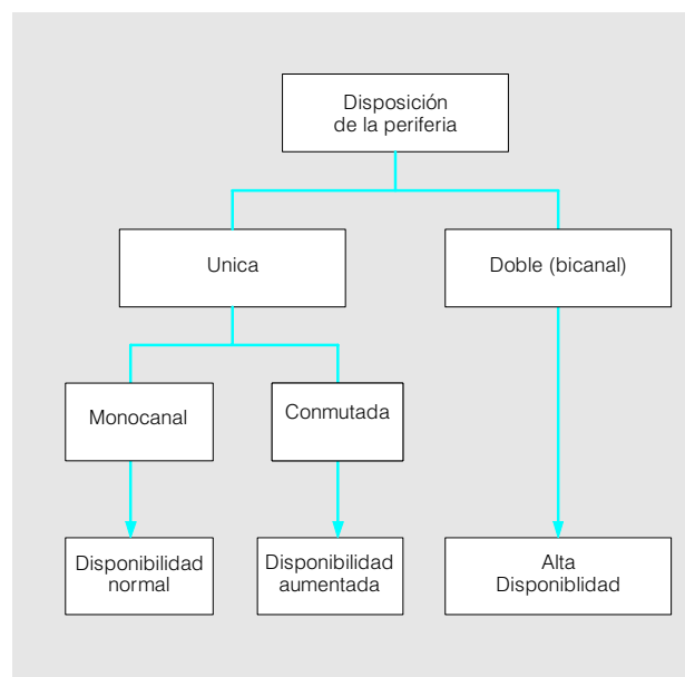
Fig. 3/8 Niveles de disponibilidad de la periferia
