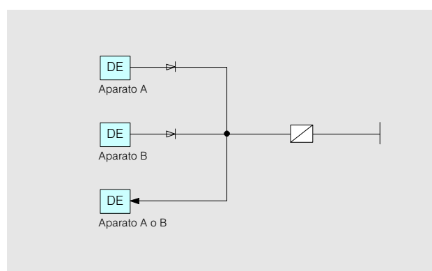
Fig. 11/3 Salida digital intermitente redundante con localización de averías
