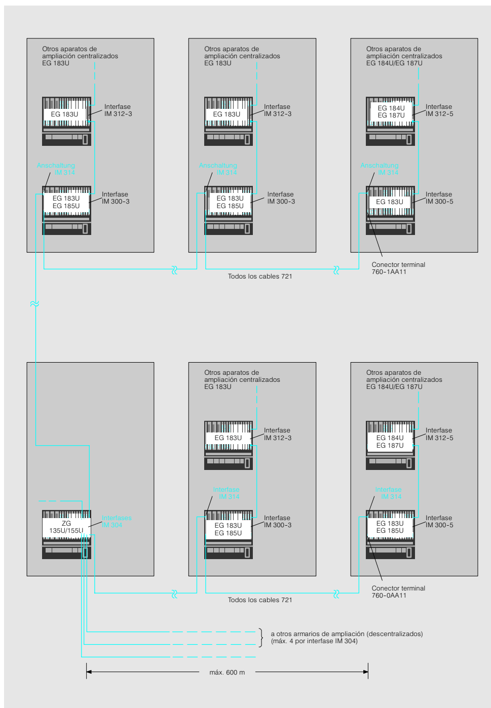
Fig. 4/52 Conexión descentralizada de aparatos de ampliación al aparato central vía interfases IM 314 e IM 304
