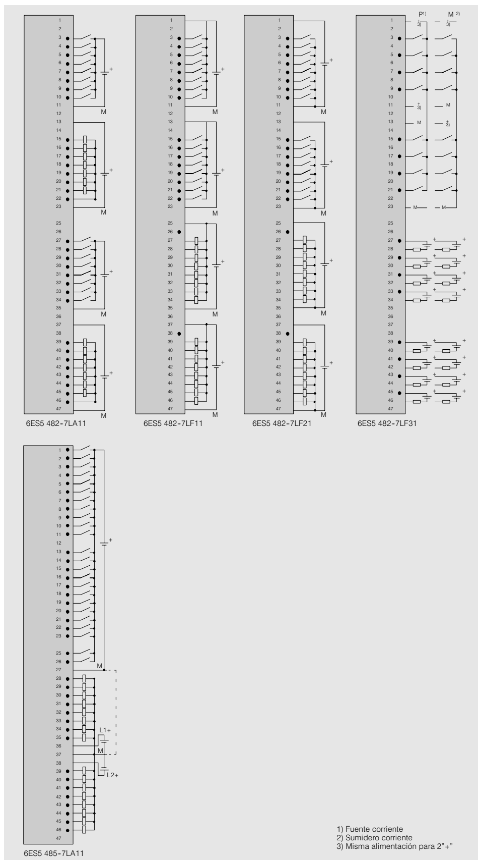
Fig. 3/29 Esquemas de conexiones para tarjetas de entrada y salida digitales
