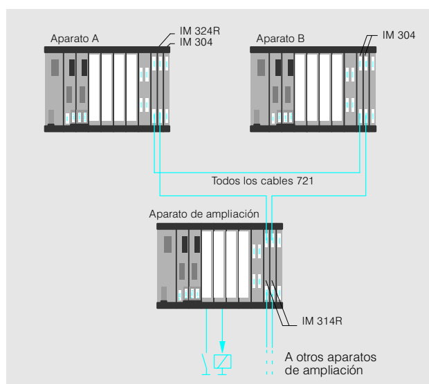
Fig. 3/10 Configuración conmutada (disponibilidad aumentada)
