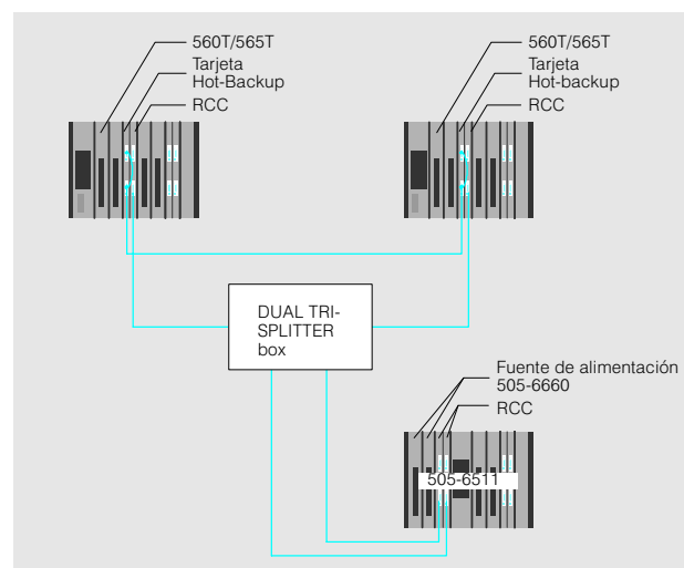
Fig. 5/3 Hot-Backup con periferia bicanal
