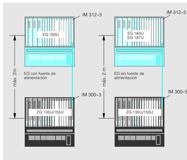
Fig. 4/2 Disposición centralizada de aparatos de ampliación
