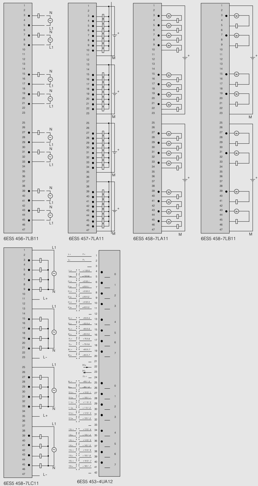
Fig. 3/28 Esquemas de conexiones para tarjetas de salida digital
