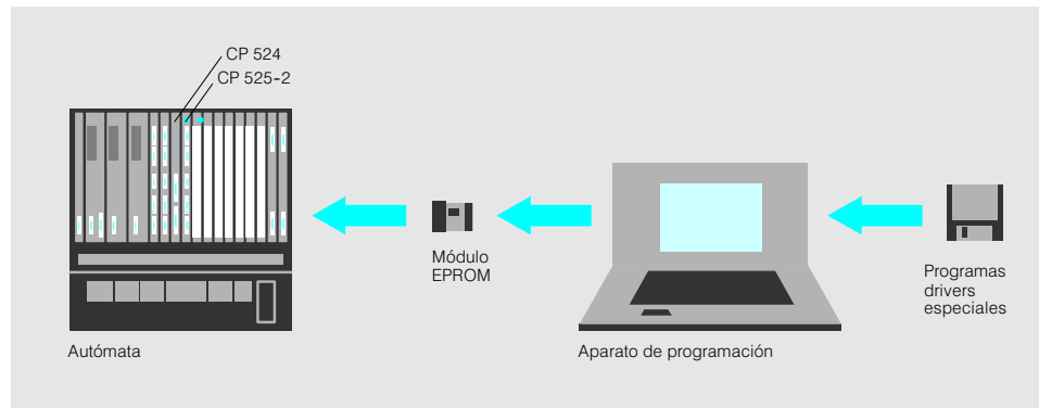
Fig. 7/89 Los programas drivers especiales en el CP 524 y CP 525-2 (driver en disquete, rutinas en EPROM para CP 524 y en EPROM o RAM para CP 525-2) son el requisito previo para el acoplamiento de sistemas terceros, tales como ordenadores u otros subsistemas (p. ej., básculas o lectores de código de barras).
