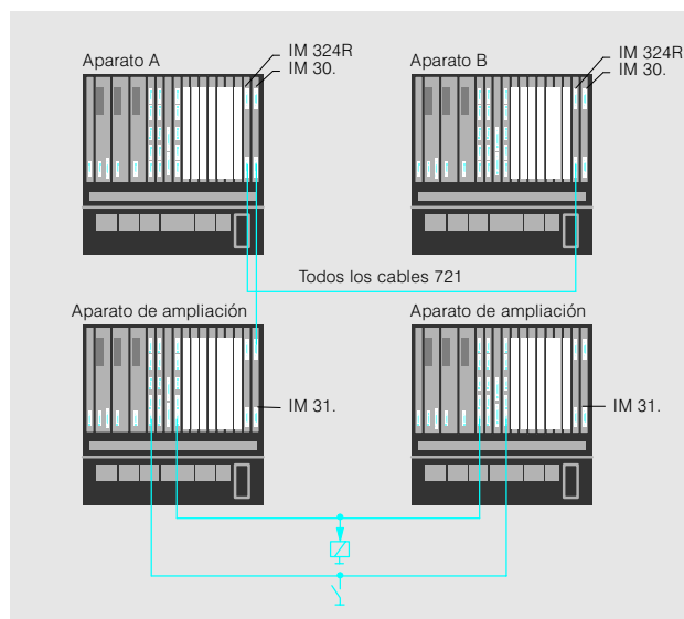
Fig. 4/16 Configuración bicanal (alta disponibilidad)
