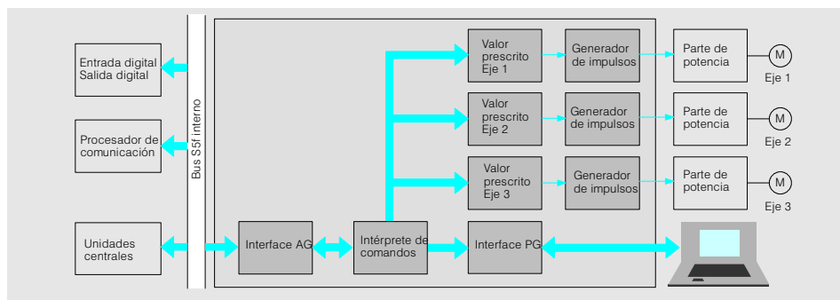
Fig. 4/36 Esquema funcional de la tarjeta IP 247
