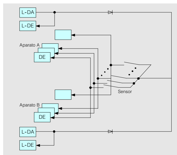
Fig. 11/2 Entrada digital redundante con localización de averías
