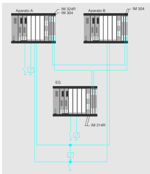
Fig. 3/12 Configuración mixta de un S5-115H
