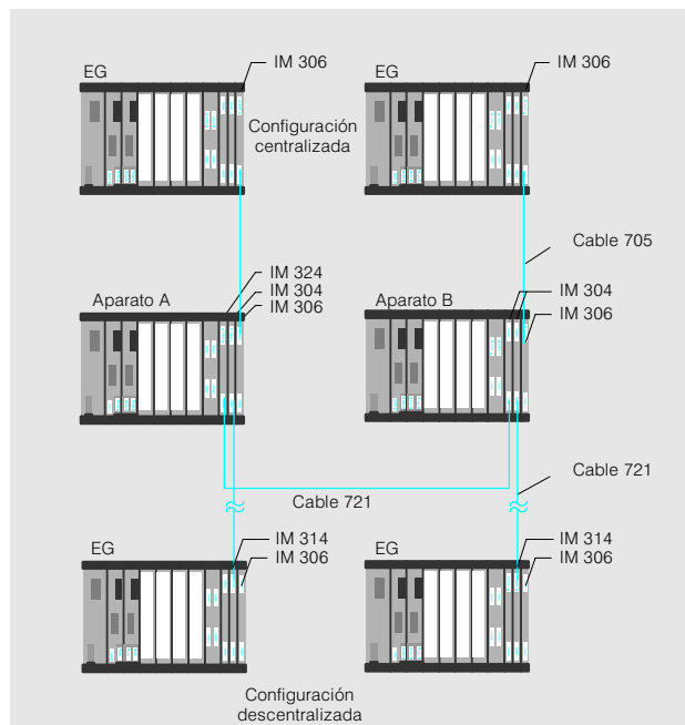
Fig. 3/18 Disp. bicanal (redundante) de la periferia (segura contra averías)
