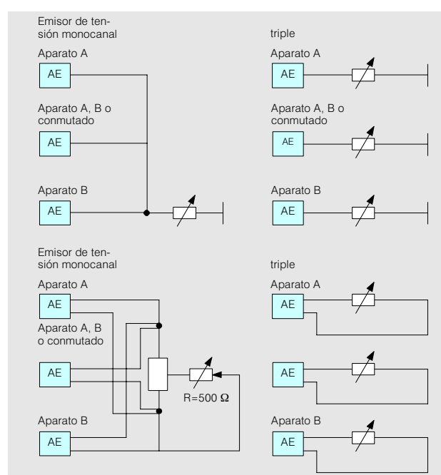
Fig. 11/12 Tarjeta analógica redundante triple
