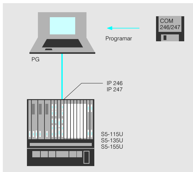
Fig. 7/14 Conexión y programación de las tarjetas de posicionamiento IP 246 e IP 247
