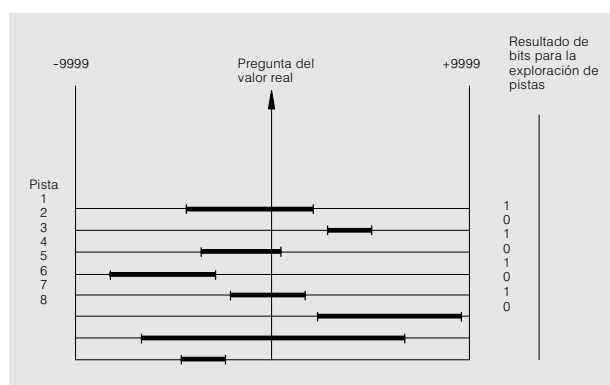
Fig. 4/29 Diagrama para un captador de recorrido
