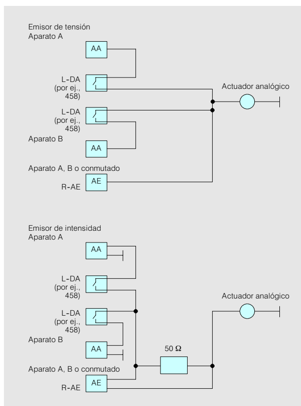
Fig. 11/13 Salidas analógicas redundantes
