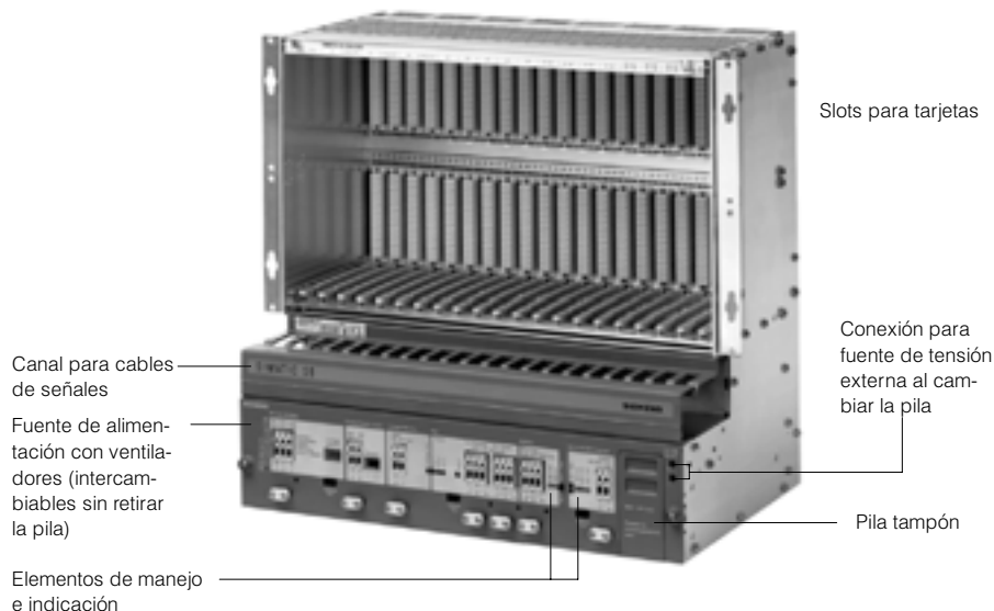
Fig. 4/4 Disposición mecánica del aparato central ZG 135U/155U para los autómatas S5-135U y S5-155U
