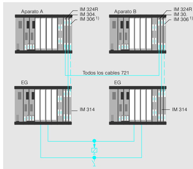
Fig. 3/11 Configuración redundante (alta disponibilidad)
