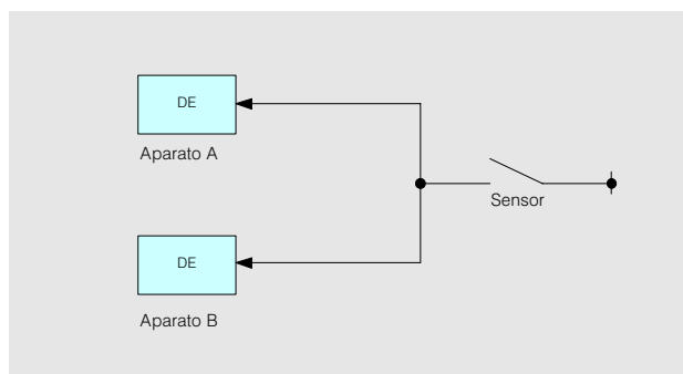
Fig. 11/6 Entrada digital redundante bicanal sin localización de fallos
