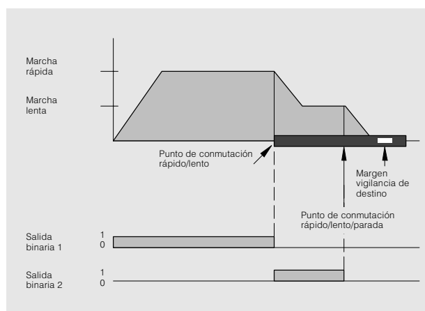
Fig. 4/30 Posicionamiento de un motor de polos conmutables
