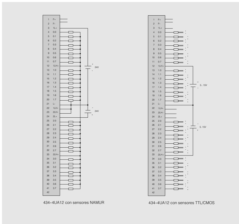
Fig. 3/26 Esquemas de conexiones para tarjetas de entrada digitales
