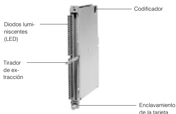
Fig. 4/5 Construcción de las tarjetas de entrada y salida
