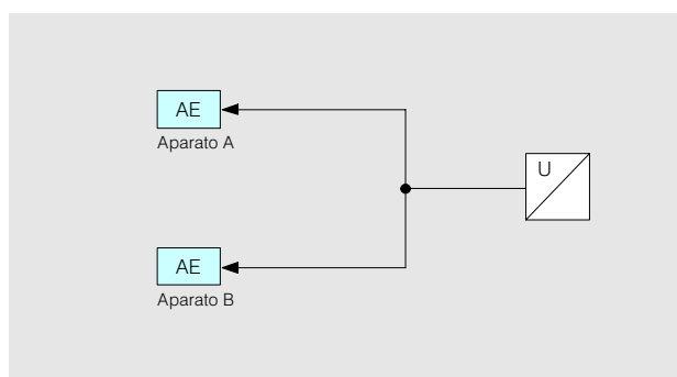
Fig. 11/5 Entrada analógica redundante
