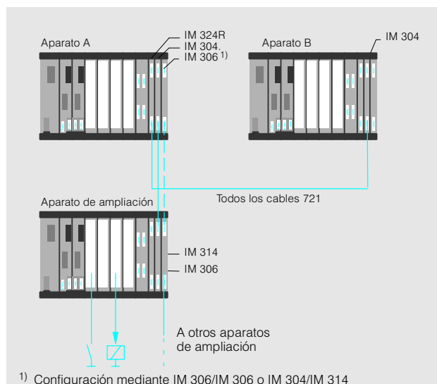
Fig. 3/9 Configuración monocanal (disponibilidad normal)
