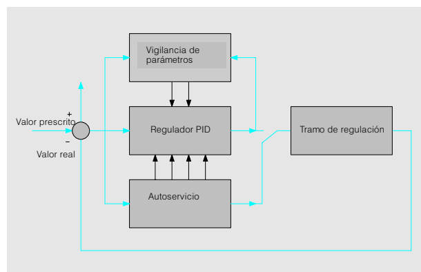
Fig. 4/34 Esquema funcional del autoajuste del regulador
