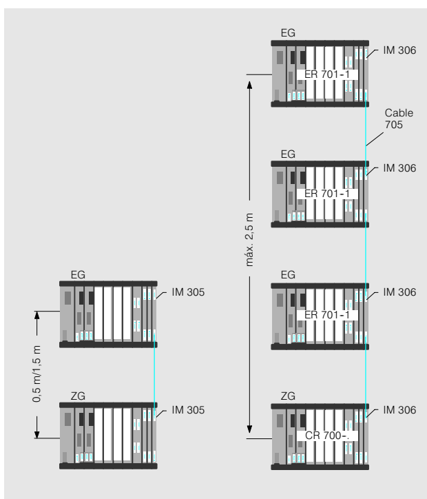
Fig. 3/33 Conexión centralizada de aparatos de ampliación a uno central por medio de las interfases IM 305 (izquierda) e IM 306 (derecha)
