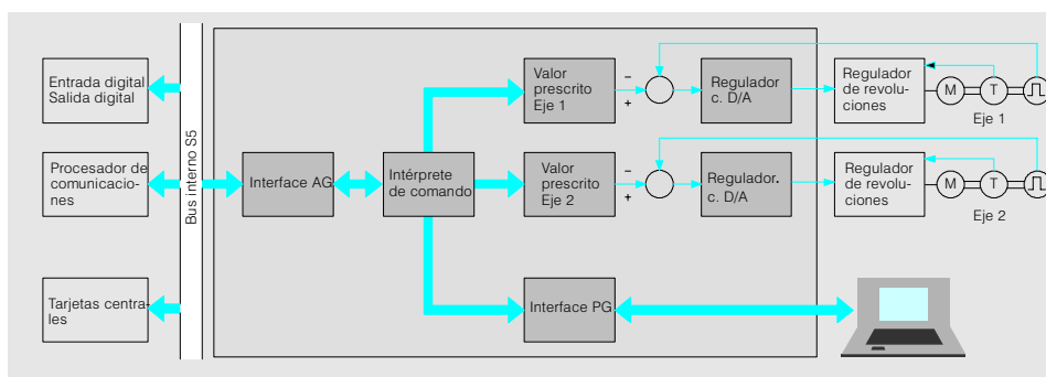
Fig. 4/35 Esquema funcional de la tarjeta IP 246
