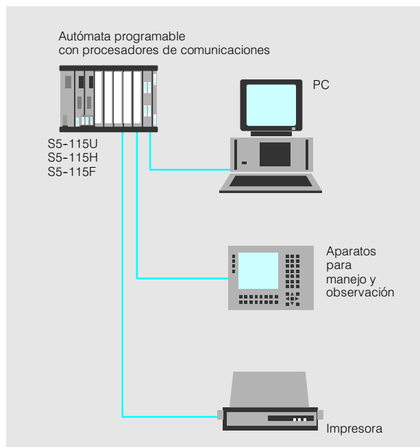
Fig. 3/6 Acoplamiento del autómata con PC, con aparatos para manejo y observación y con impresoras.
