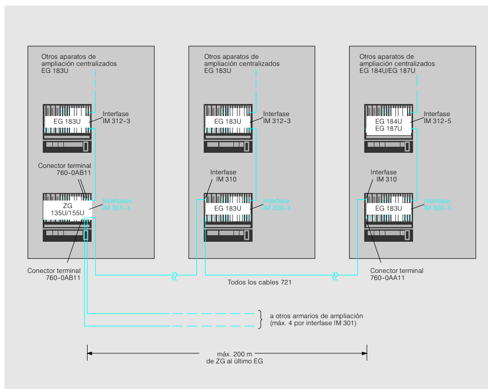
Fig. 4/50 Conexión descentralizada de EG 183U al aparato central vía interfases IM 310 e IM 301-3
