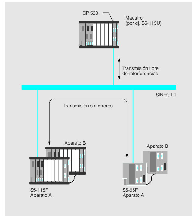
Fig. 3/23 Acoplamiento monocanal seguro
