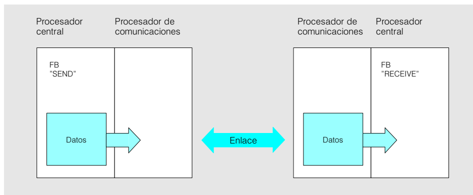
Fig. 7/88 Ejemplo de transmisión de datos usando módulos de manipulación
