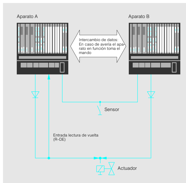
Fig. 4/21 Configuración redundante bicanal de IP/CP
