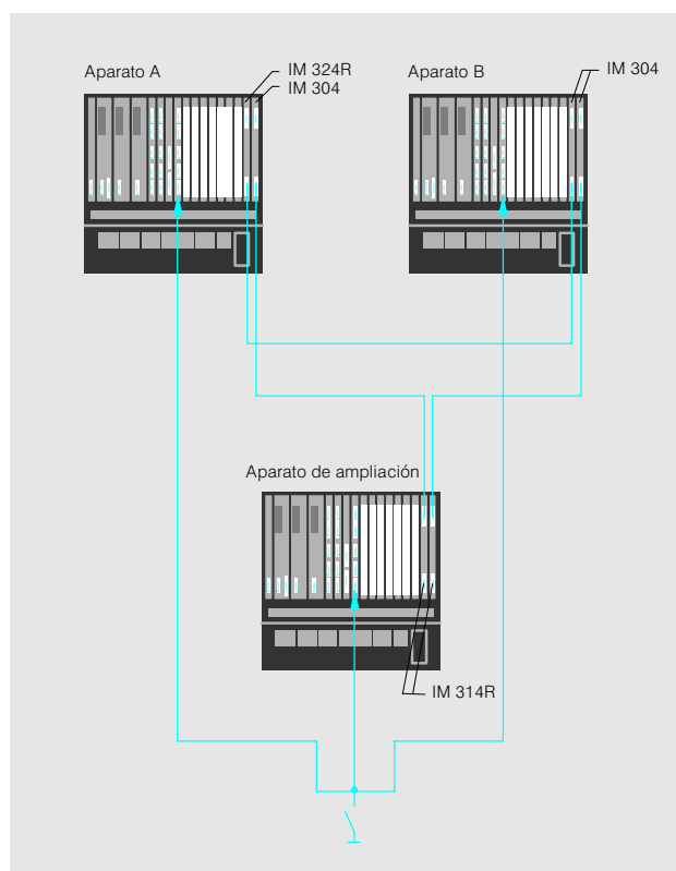
Fig. 4/17 Configuración en 3 canales (máxima disponibilidad)
