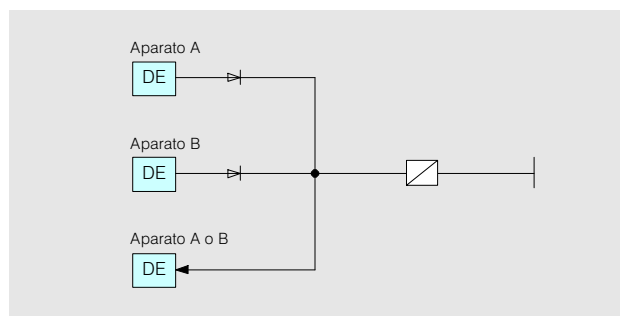
Fig. 11/9 Salida digital intermitente redundante bicanal con localización de fallos reducida
