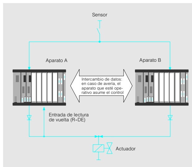
Fig. 3/14 Ejemplo de S5-115H con entrada y salida redundantes
