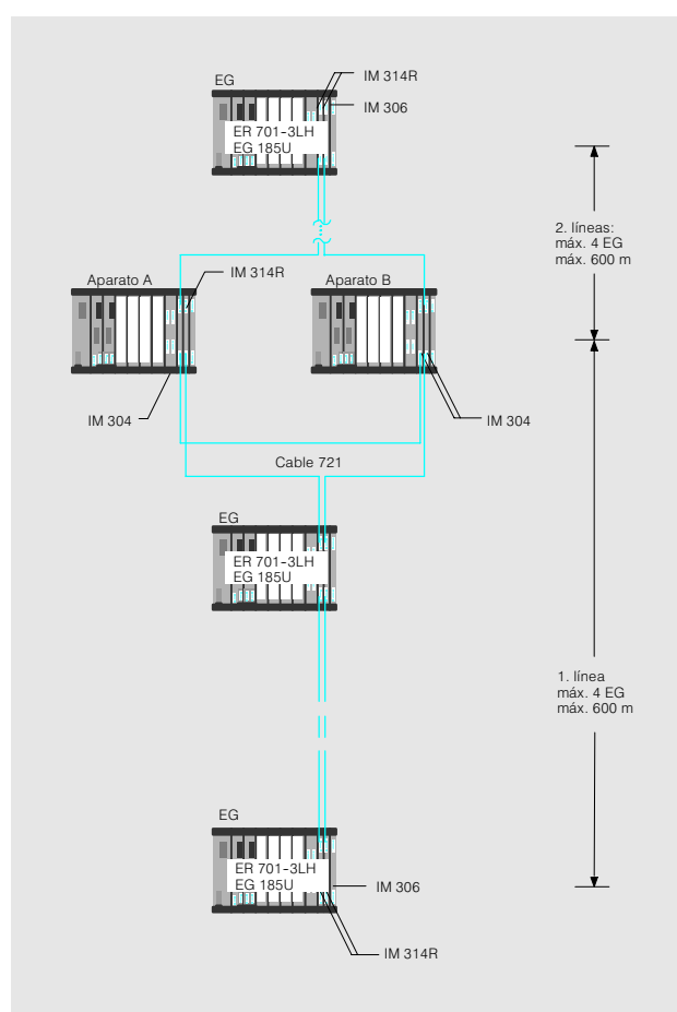
Fig. 3/38 Configuración conmutada descentralizada de tarjetas periféricas
