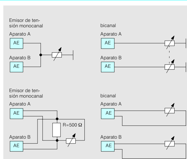
Fig. 11/11 Entradas analógicas redundantes bicanales
