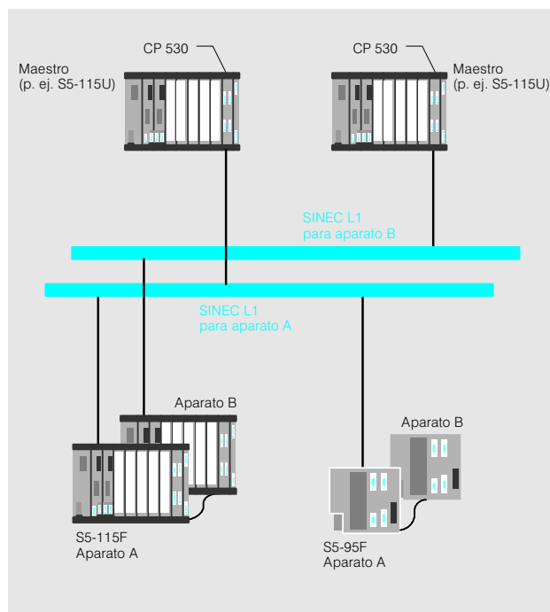
Fig. 3/24 Acoplamiento de seguridad bicanal
