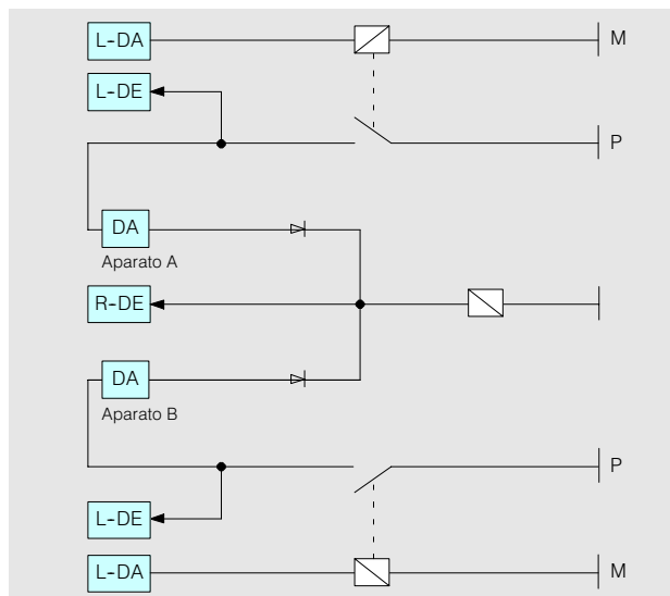
Fig. 11/4 Salida digital intermitente redundante con localización de averías limitada
