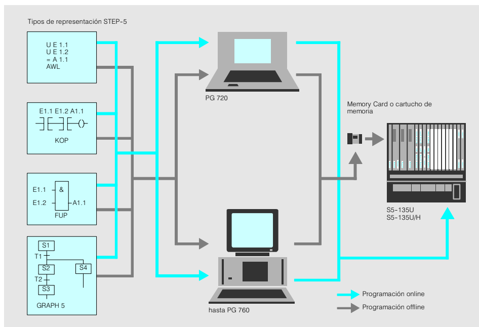
Fig. 4/10 Programación del S5-135U y S5-155U/H
