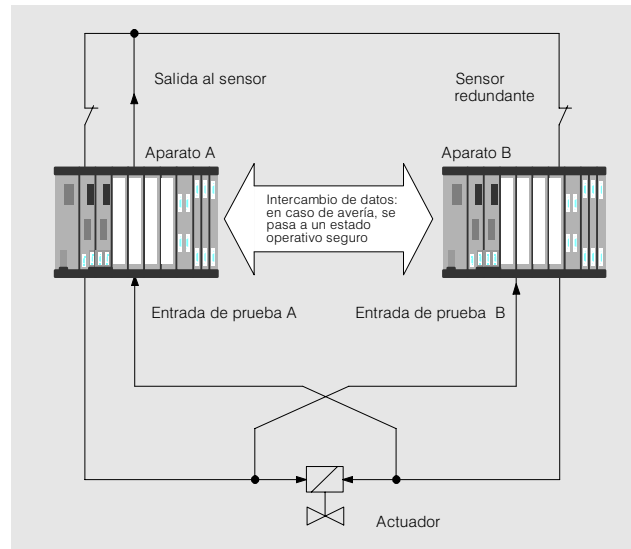
Fig. 3/20 Ejemplo de S5-115F con entradas y salidas seguras
