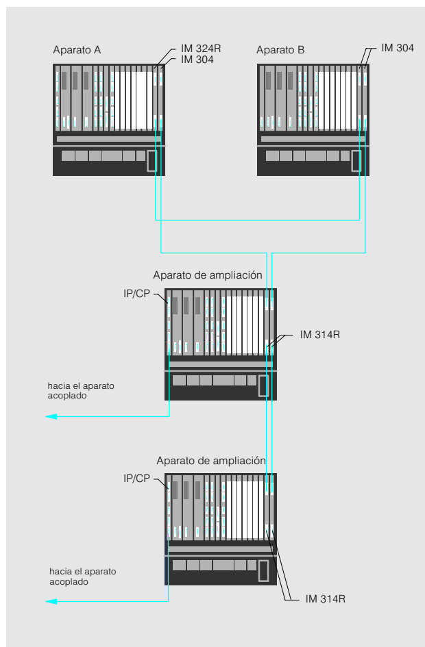
Fig. 4/19 Configuración redundante conmutada de IP/CP
