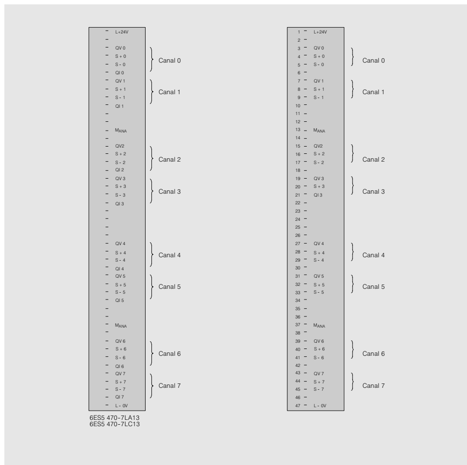
Fig. 3/32 Esquemas de conexiones para tarjetas de salida analógica
