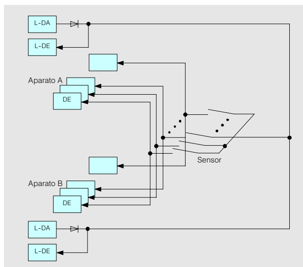
Fig. 11/7 Entradas digitales redundantes bicanales con localización de fallos
