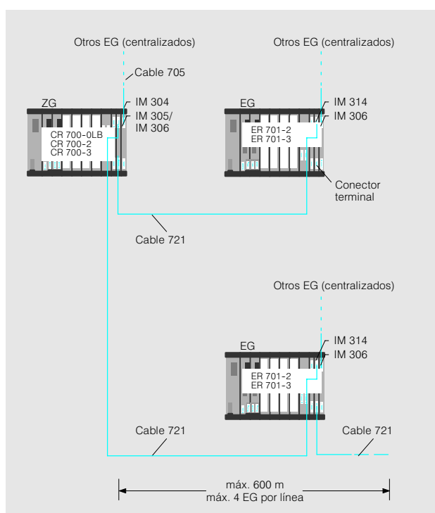
Fig. 3/34 Conexión descentralizada de aparatos de ampliación a uno central por medio de las interfases IM 304 e IM 314
