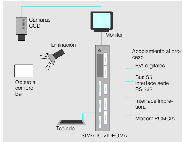
Fig. 4/45 Sistema de visión artificial SIMATIC VIDEOMAT
