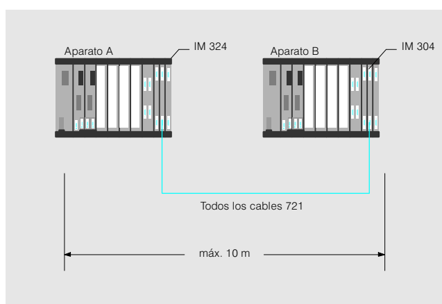
Fig. 3/39 Acoplamiento de los aparatos centrales
