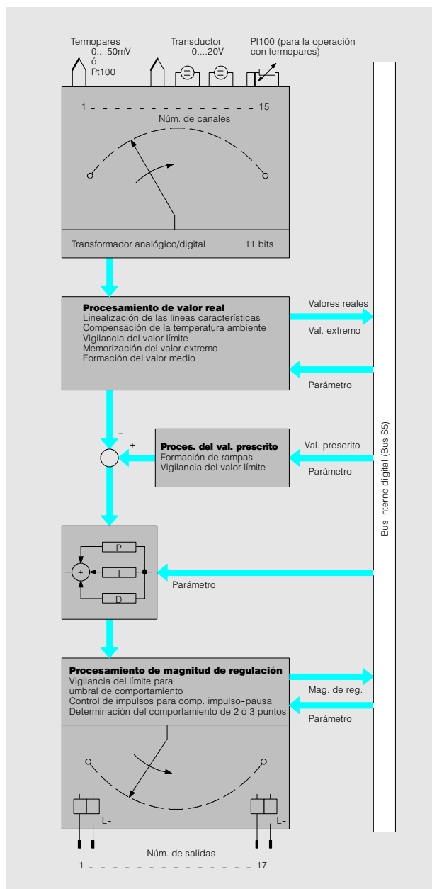
Fig. 4/33 Esquema funcional de la tarjeta de regulación de temperatura
