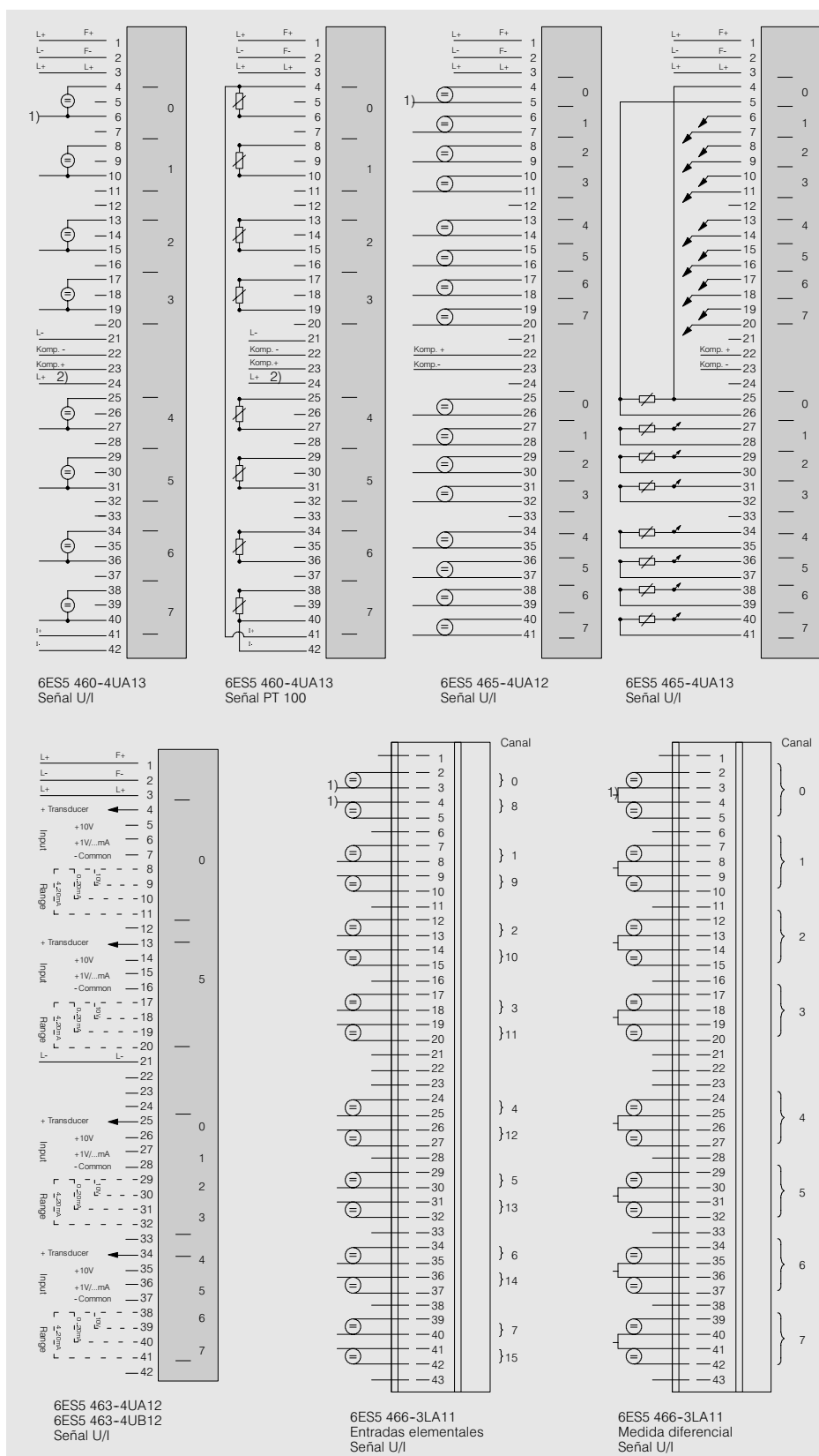
Fig. 4/26 Esquema de conexiones para tarjetas de entrada analógica
