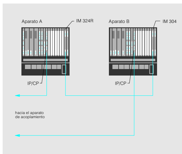
Fig. 4/20 Configuración redundante bicanal CP/IP
