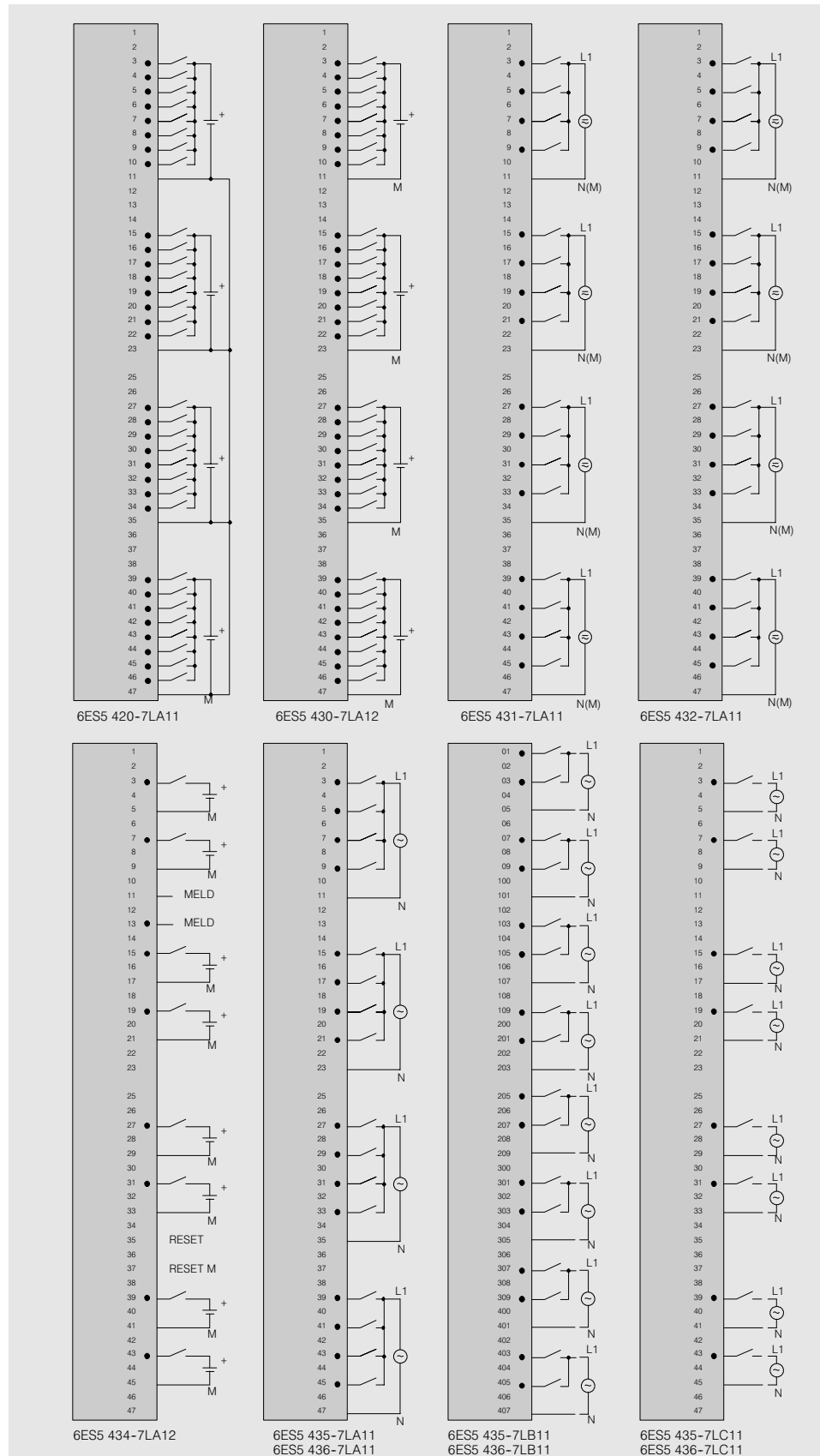
Fig. 3/25 Esquemas de conexiones para tarjetas de entrada digitales
