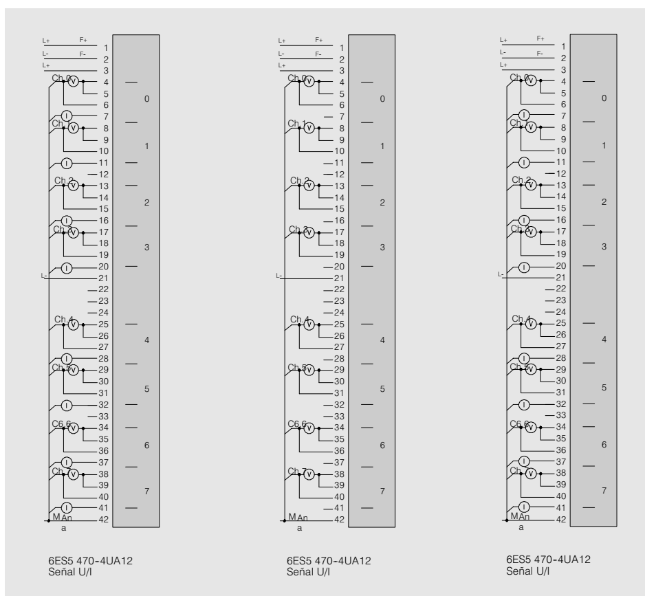
Fig. 4/27 Esquemas de conexión para tarjetas de salida analógica
