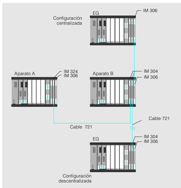
Fig. 3/19 Disposición monocanal de la periferia (segura en el aparato central, no segura en el de ampliación)
