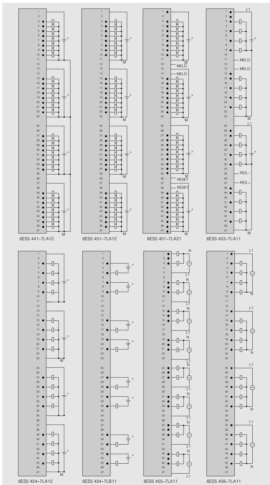
Fig. 3/27 Esquemas de conexiones para tarjetas de salida digital
