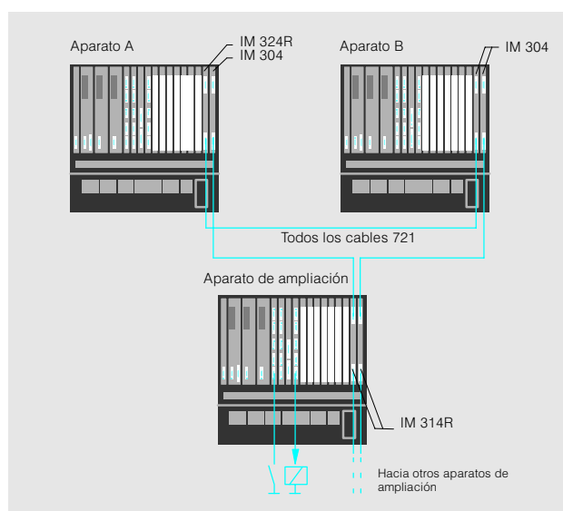
Fig. 4/15 Configuración conmutada (disponibilidad aumentada)
