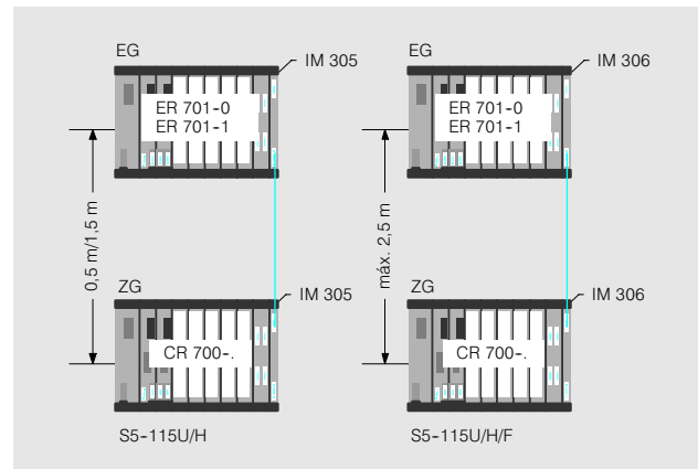
Fig. 3/2 Conexión centralizada de aparatos de ampliación
