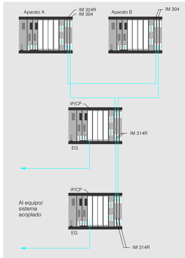
Fig. 3/13 Configuración redundante conmutada de IP/CP
