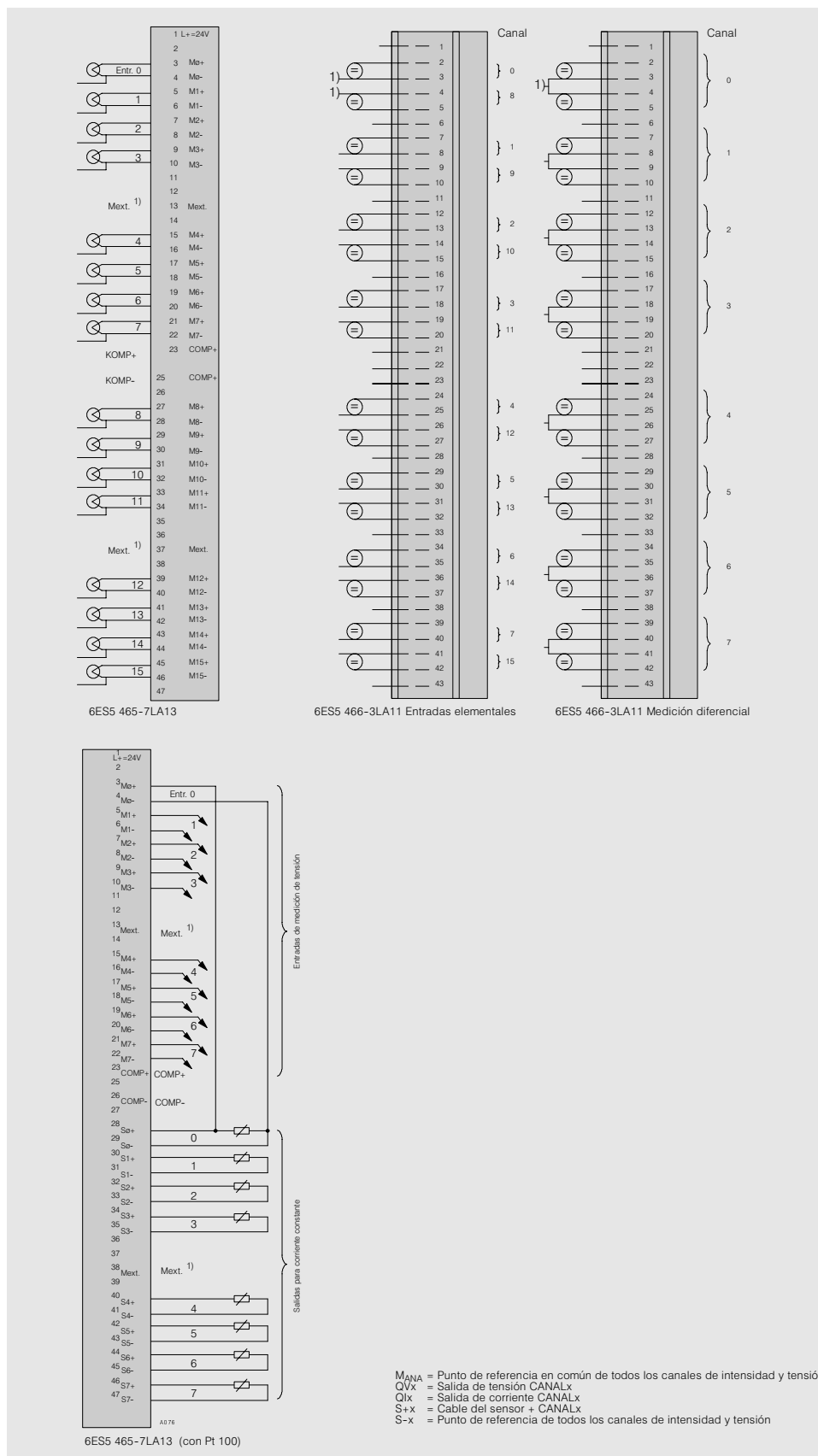
Fig. 3/31 Esquemas de conexiones para tarjetas de entrada analógica
