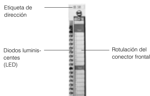
Fig. 4/7 Tarjetas de entrada/salida con tiras rotulables
