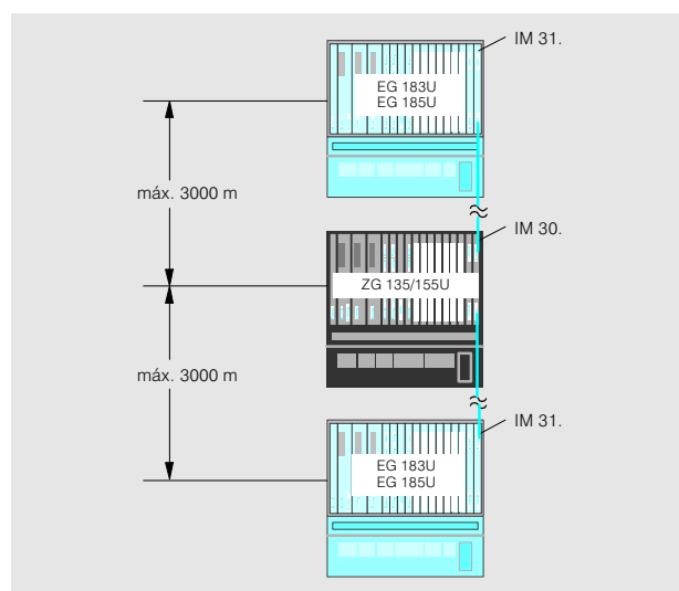
Fig. 4/3 Disposición descentralizada de aparatos de ampliación
