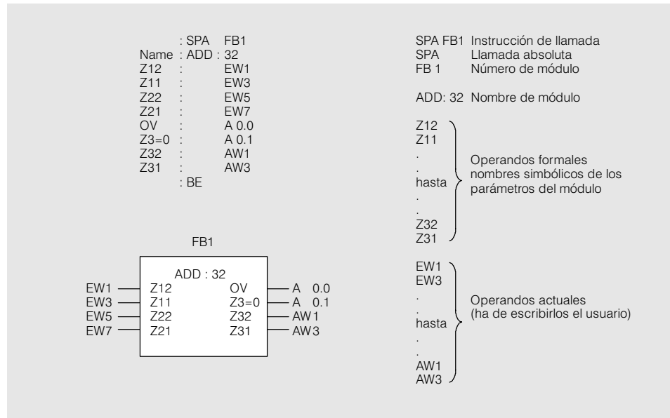
Fig. 7/29 Representación de módulos funcionales estándar en el aparato de programación arriba: como lista de instrucciones (AWL) abajo: como esquema de funciones (FUP)
