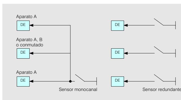
Fig. 11/8 Entrada digital redundante triple
