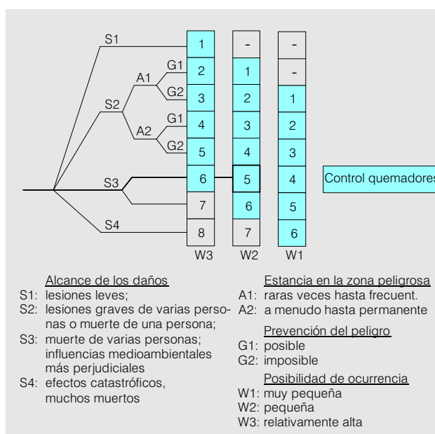
Fig. 3/17 Grafo de riesgo para las categorías de seguridad según DIN V 19250 con dos ejemplos
