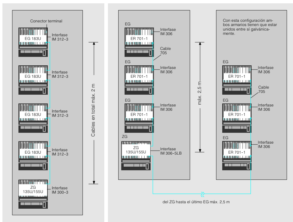
Fig. 4/47 Conexión centralizada de aparatos de ampliación con fuente de alimentación insertada en el aparato central vía interfases IM 312-3 e IM 300-3.
