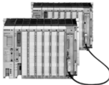
Fig. 3/7 Autómata S5-115H
