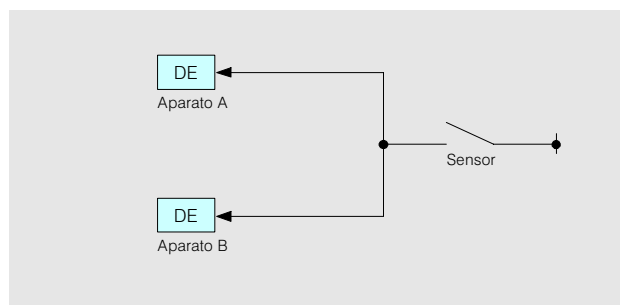
Fig. 11/1 Entrada digital redundante sin localización de averías
