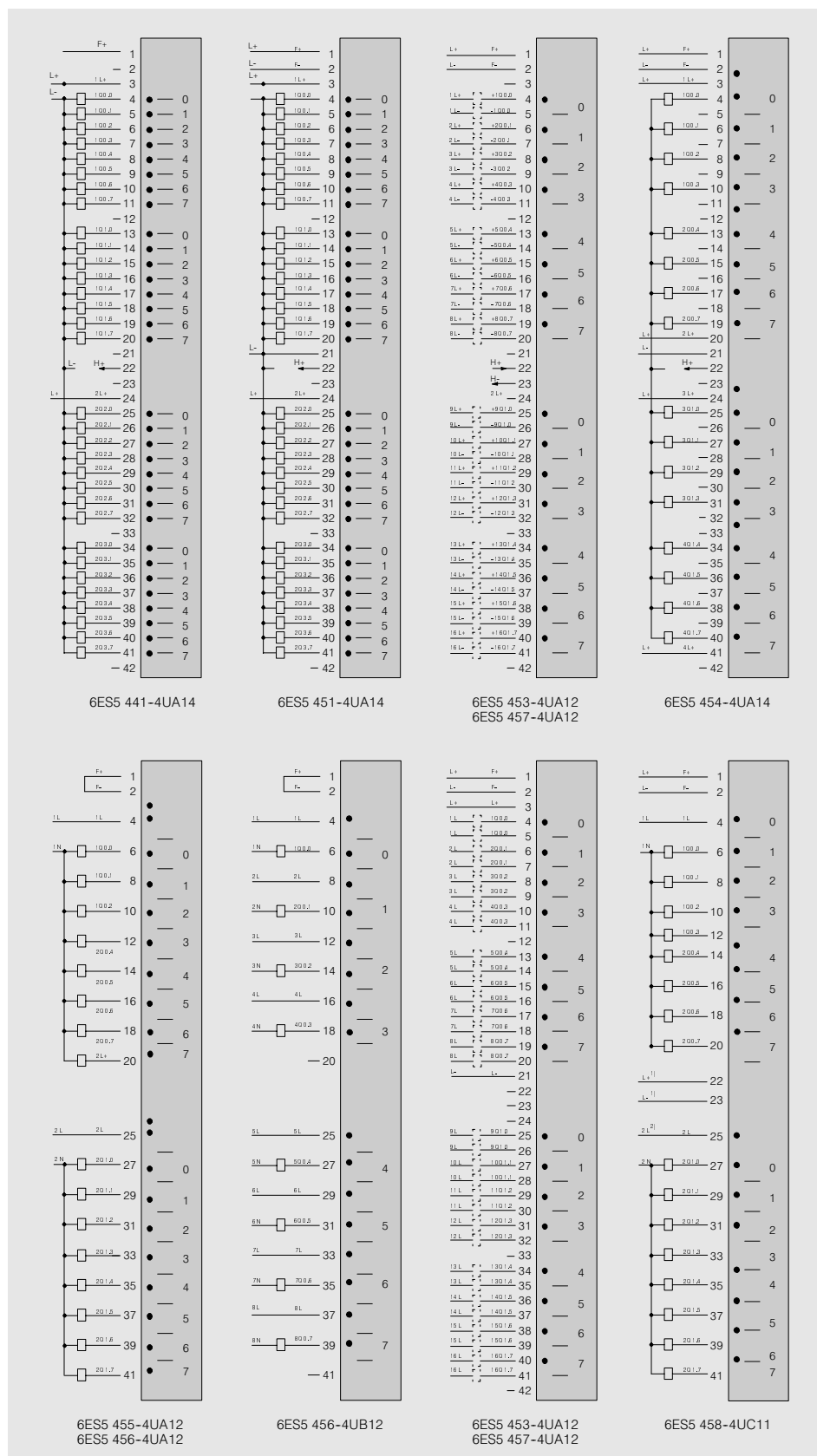
Fig. 4/24 Esquema de conexiones de las tarjetas de salida digital
