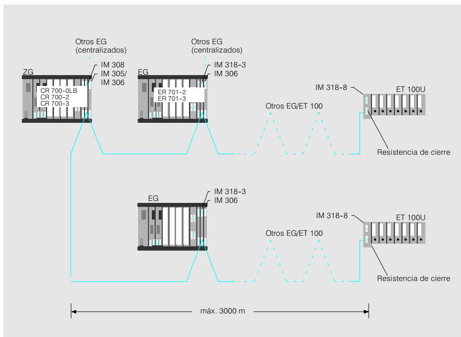
Fig. 3/36 Conexión descentralizada de aparatos de ampliación y regletas electrónicas ET 100U a un aparato central por medio de las interfases IM 308 e IM 318
